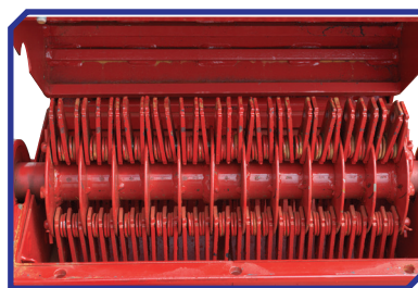
Triturador 202 - rotor com 54 martelos oscilantes.
